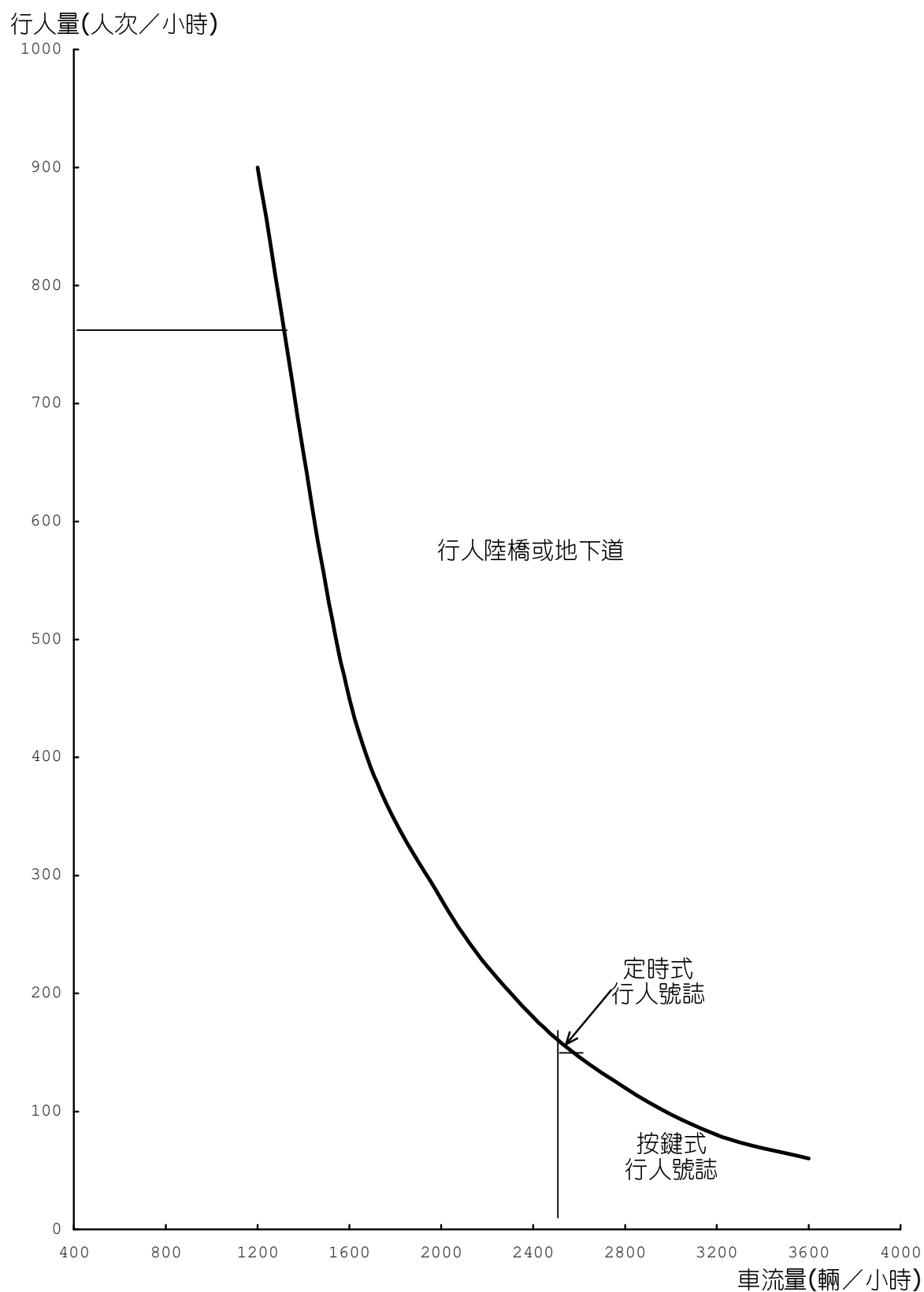
圖 3-7 各式行人穿越之設置標準(30 公尺，單元 3)
