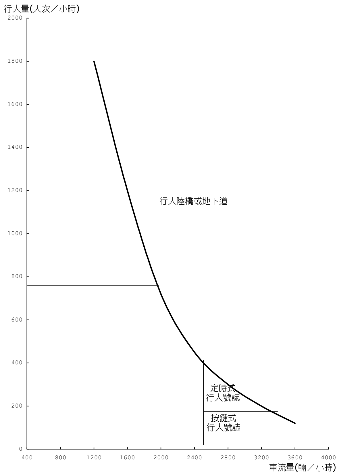
圖 3-6 各式行人穿越之設置標準(30 公尺，單元 2)
