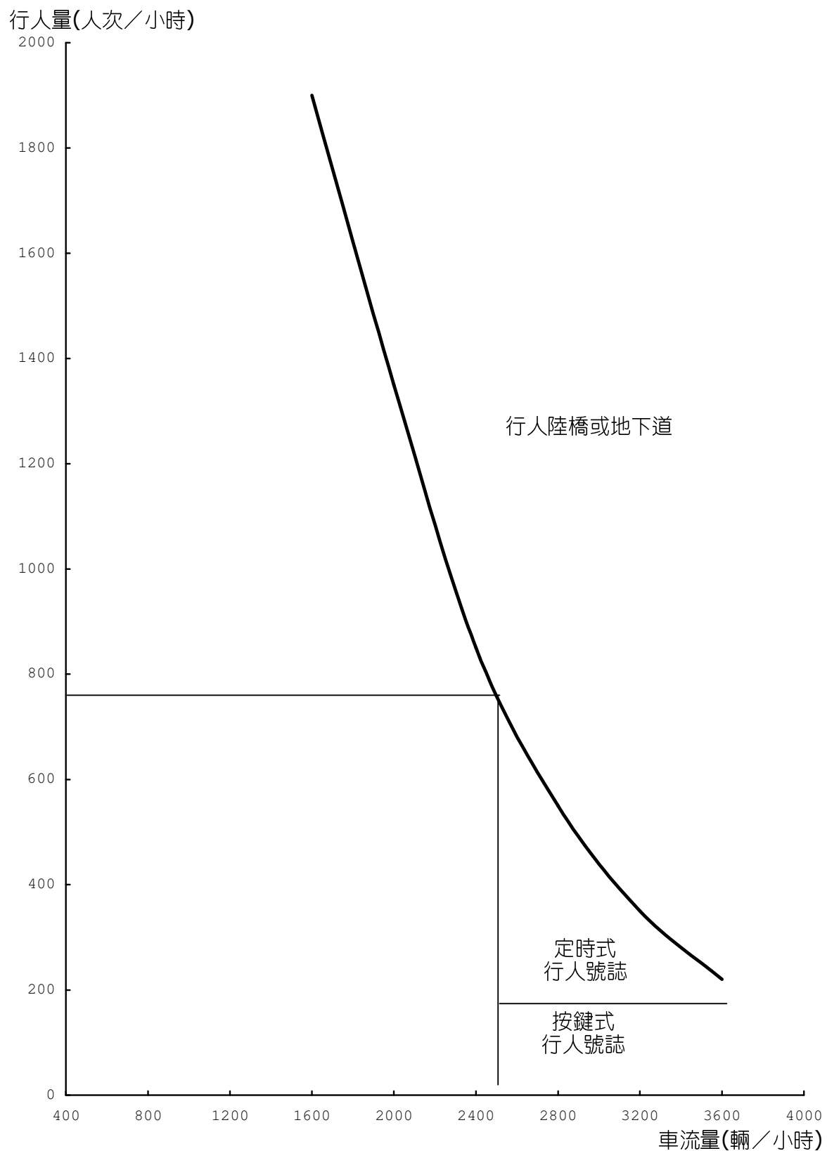
圖 3-5 各式行人穿越之設置標準(30 公尺，單元 1)
