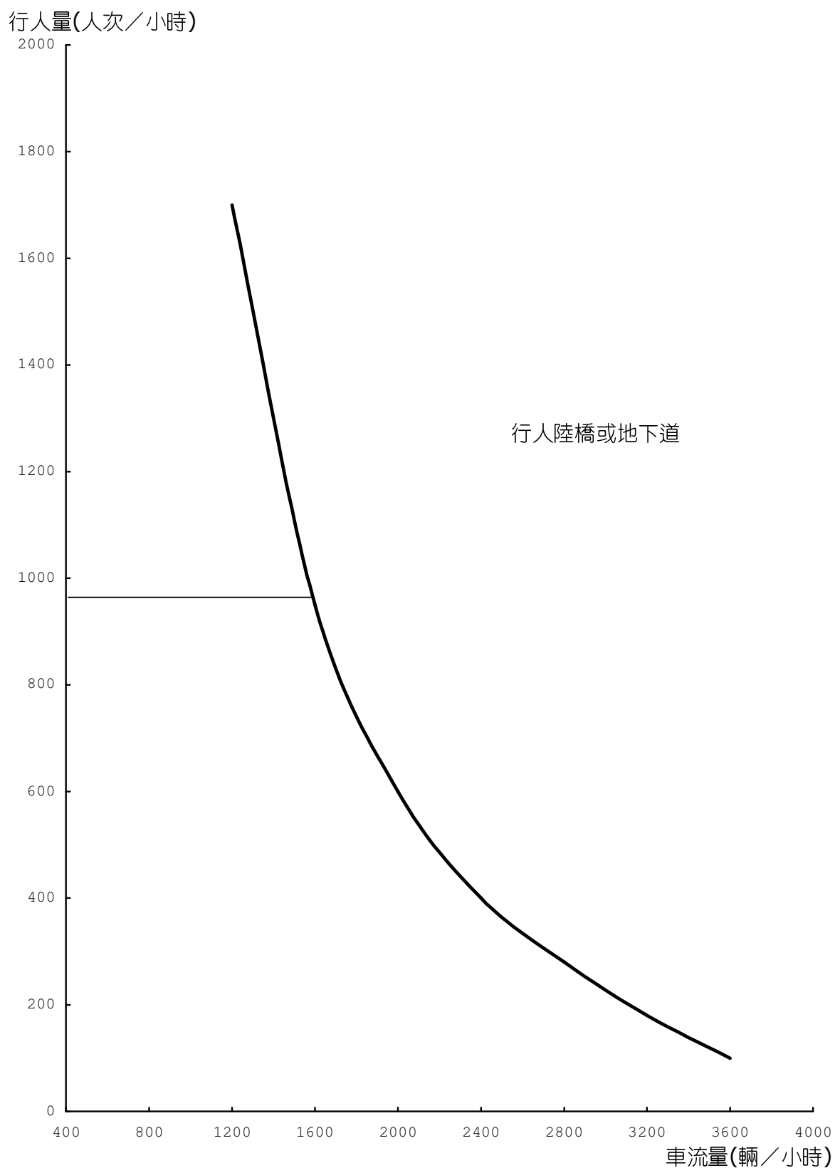
圖 3-3 各式行人穿越之設置標準(20 公尺，單元 2)
