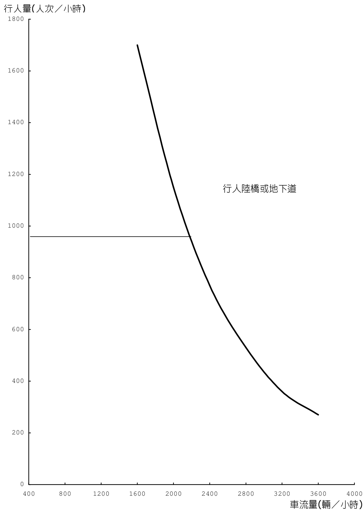
圖 3-2 各式行人穿越之設置標準(20 公尺，單元 1)
