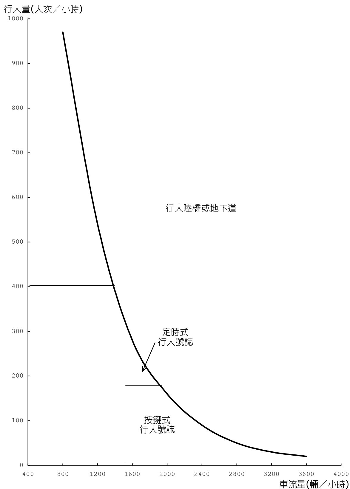
圖 3-13 各式行人穿越之設置標準(60 公尺，單元 3)
