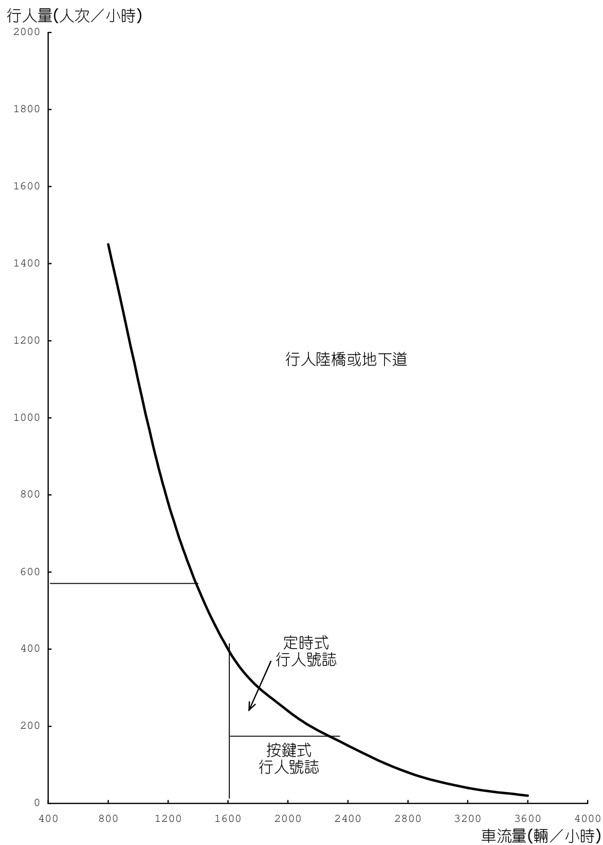
圖 3-9 各式行人穿越之設置標準(40 公尺，單元 2)
