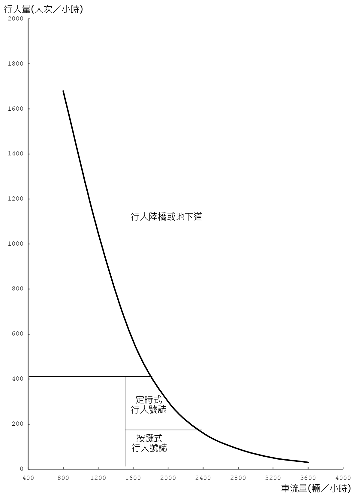
圖 3-12 各式行人穿越之設置標準(60 公尺，單元 2)
