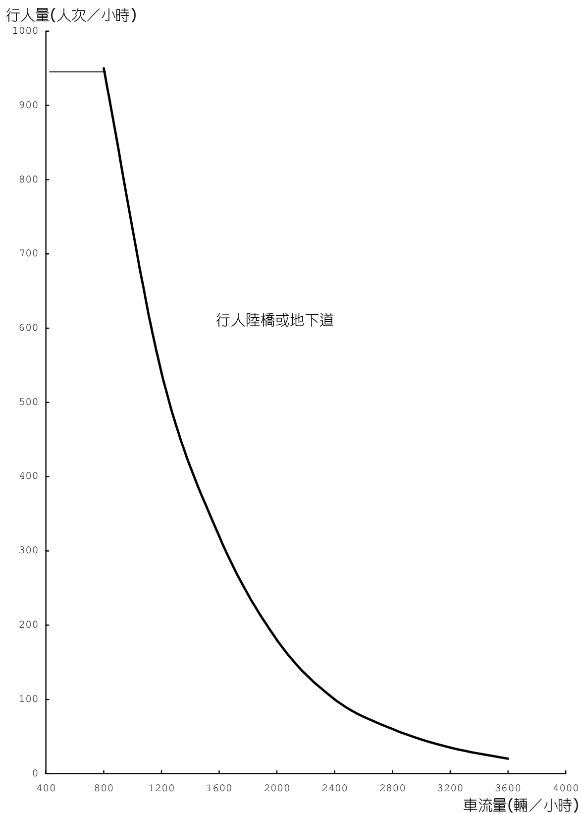
圖 3-4 各式行人穿越之設置標準(20 公尺，單元 3)
