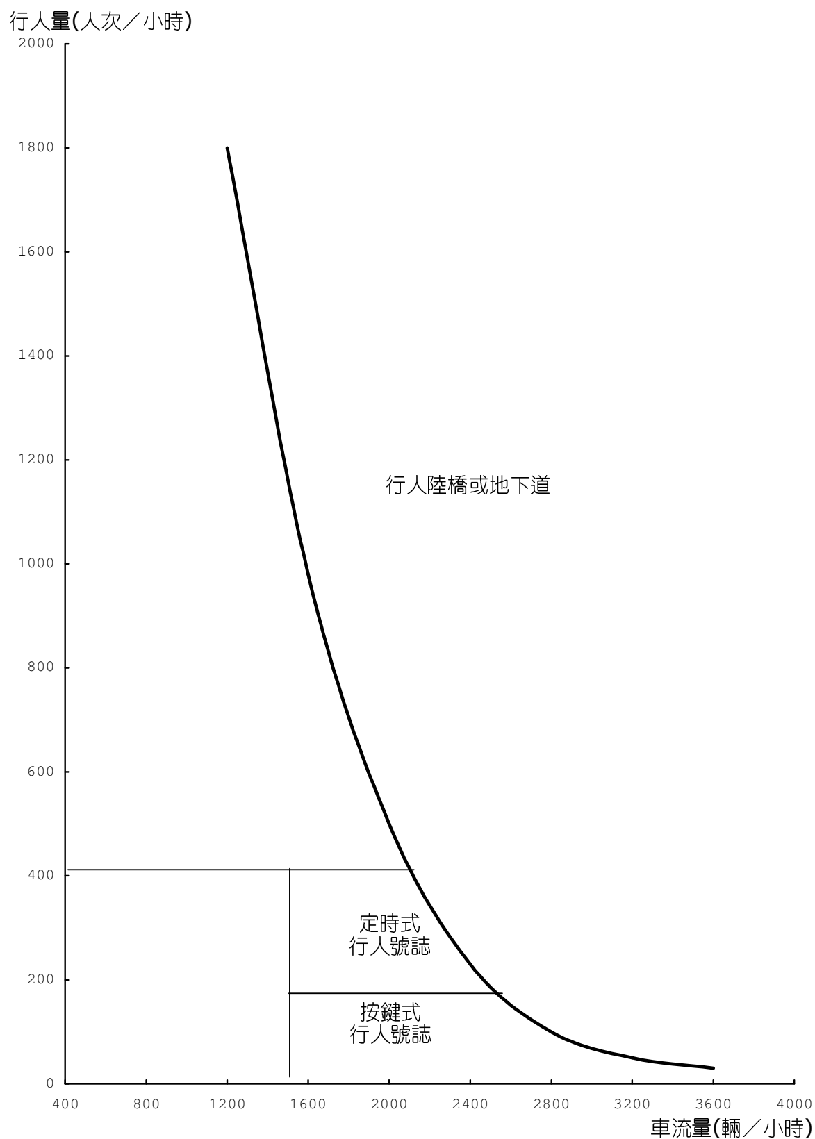
圖 3-11 各式行人穿越之設置標準(60 公尺，單元 1)
