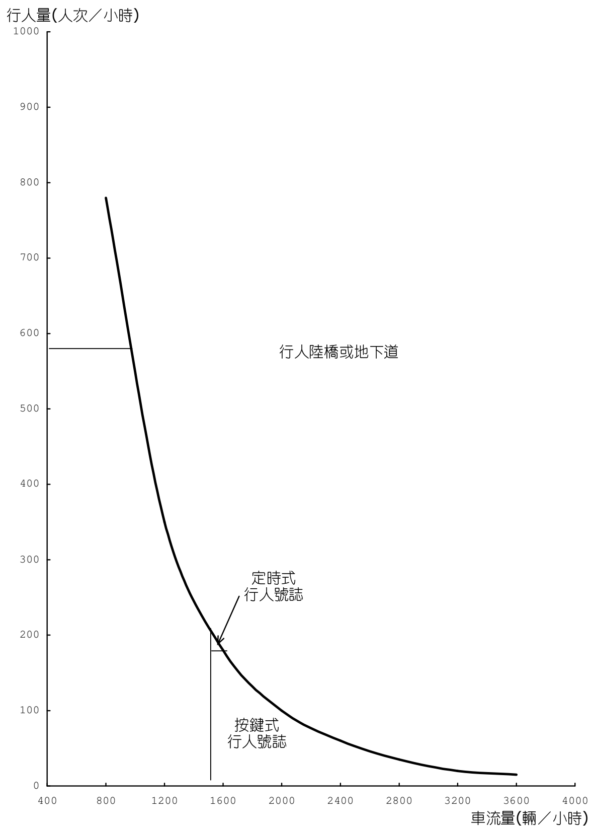
圖 3-10 各式行人穿越之設置標準(40 公尺，單元 3)
