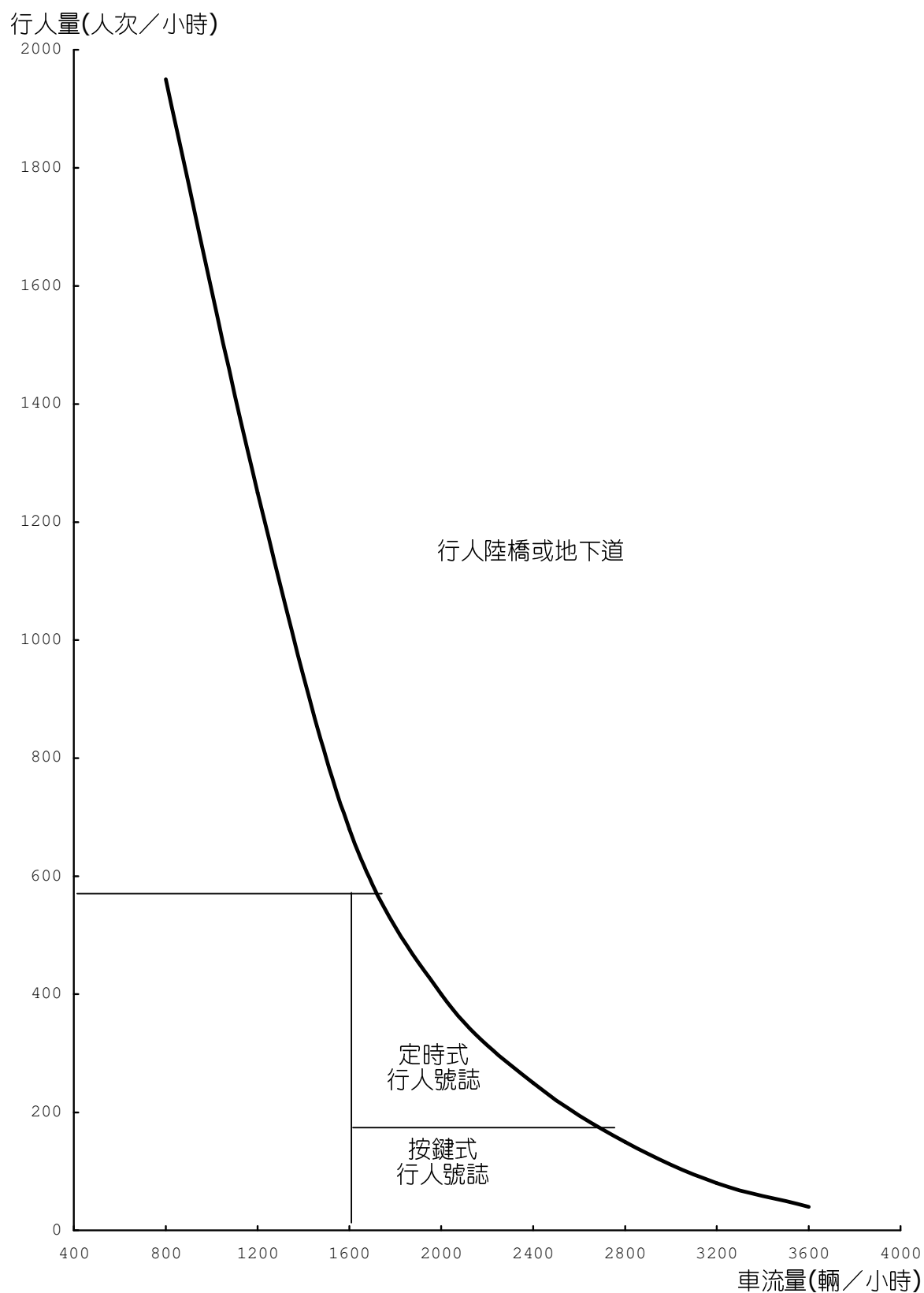
圖 3-8 各式行人穿越之設置標準(40 公尺，單元 1)
